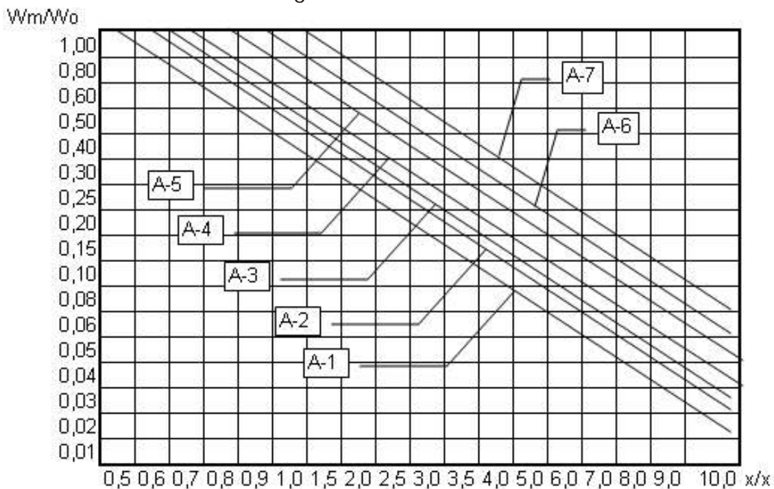
Zasięgi strumieni anemostatu
