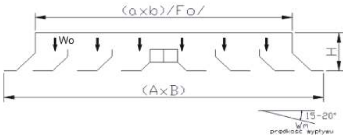
Zasięgi strumieni anemostatu
